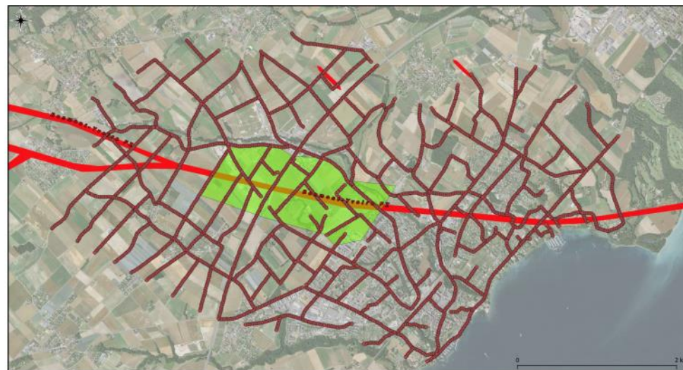
Figure 4: Faille de Bonmont-Yvoire visée par la nouvelle sismique 3D. Les points rouges représentent les points de vibration. La zone surlignée correspond à la zone d'intérêt pour un potentiel forage. La faille de Bonmont Yvoire est en rouge (orientation Est-Ouest).
